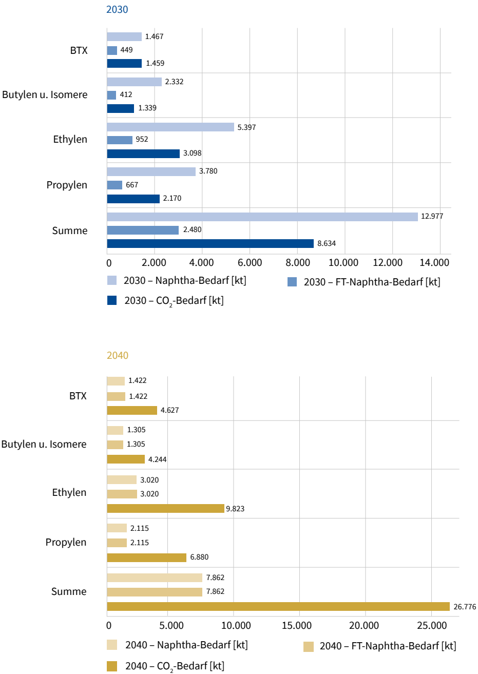
Abbildung 15: Rohstoffbedarf für Olefine und Aromaten nach Szenario 2
