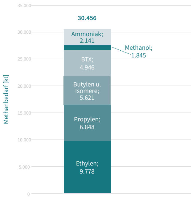
Abbildung 10: Methanbedarf für die Produktion von Grundchemikalien im Jahr 2045 mit Wasserstoff aus der Methanpyrolyse
